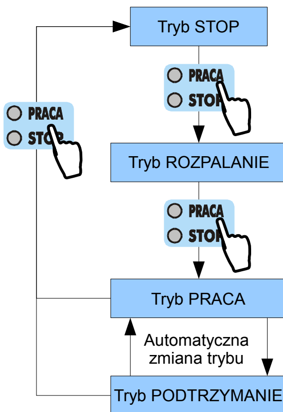
Rysunek 5: Tryby pracy regulatora i działanie klawisza PRACA/STOP.
