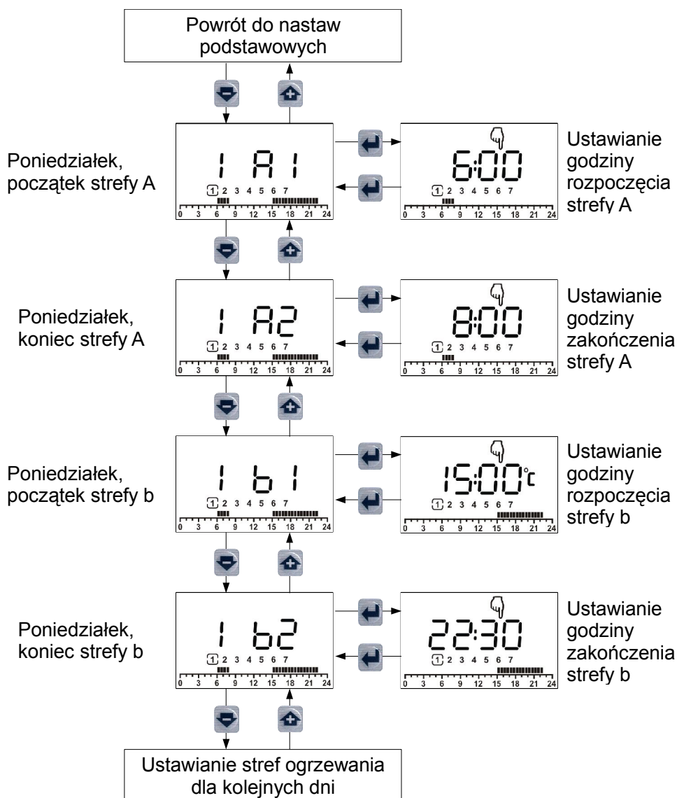
Rysunek 4: Schemat menu - ustawianie stref ogrzewania.
