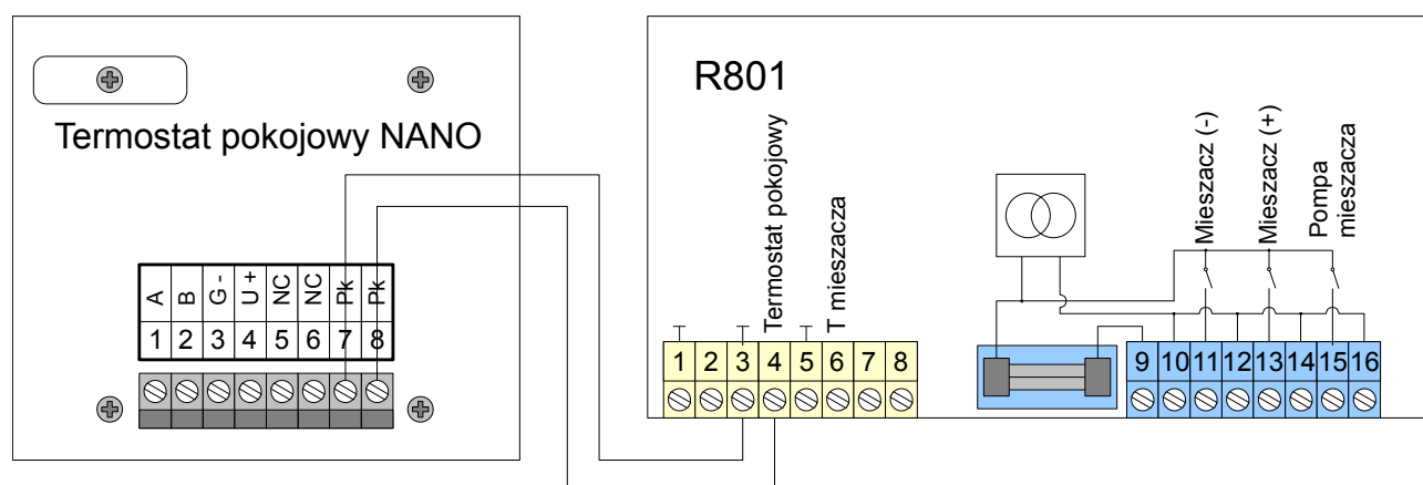
Rysunek 3: Połączenie wyjścia przekaźnikowego termostatu pokojowego NANO do regulatora mieszacza R801
