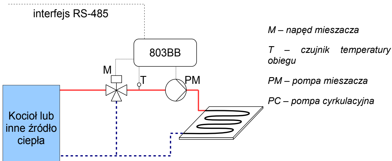
Rysunek 1: Schemat instalacji z kontrolą temperatury bufora i sterowaniem pompą PCO2
