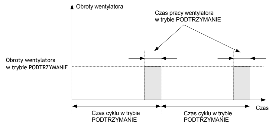
Rysunek 4: Schemat sterowania wentylatorem w trybie PODTRZYMANIE
