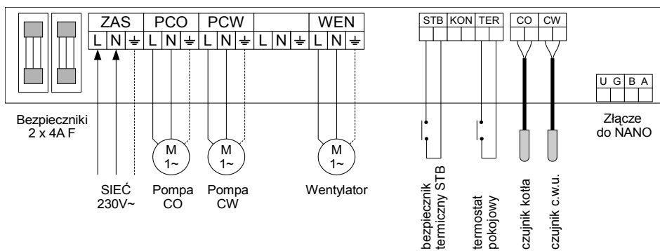
Rysunek 5: Schemat podłączenia.
