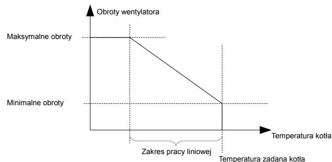
Rysunek 3: Schemat sterowania wentylatorem w trybie PRACA
