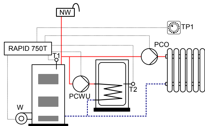
Rysunek 1: Schemat hydrauliczny układu z obsługą ciepłej wody.
