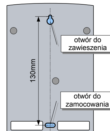
Ilustracja 3: Rozmieszczenie otworów montażowych
