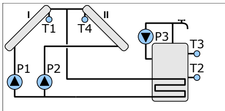
Schemat 12 Ładowanie zasobnika z dwupięciowego układu kolektorów. Sterowanie pracą dwupompowej grupy solarnej. Sterowanie pompą cyrkulacyjną.
