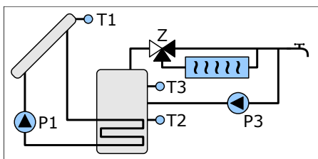
Schemat 13 Ładowanie zasobnika z kolektora słonecznego, schemat z trzema czujnikami. Sterowanie zaworem kierującym CWU przez podgrzewacz przepływu. Sterowanie pompą cyrkulacyjną.
