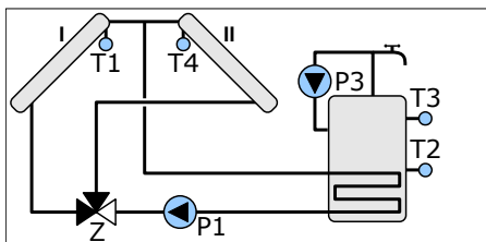
Schemat 15 Ładowanie zasobnika z dwóch kolektorów w układzie z zaworem przełączającym. Sterowanie pompą cyrkulacyjną.
