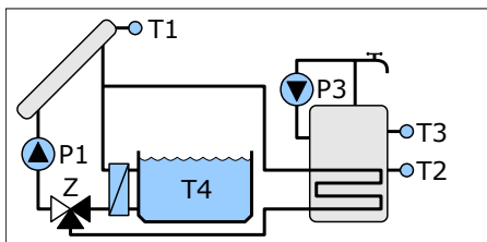
Schemat 14 Ładowanie zasobnika z kolektora słonecznego, schemat z trzema czujnikami. Sterowanie ładowaniem basenu w układzie z zaworem przełączającym. Sterowanie pompą cyrkulacyjną.
