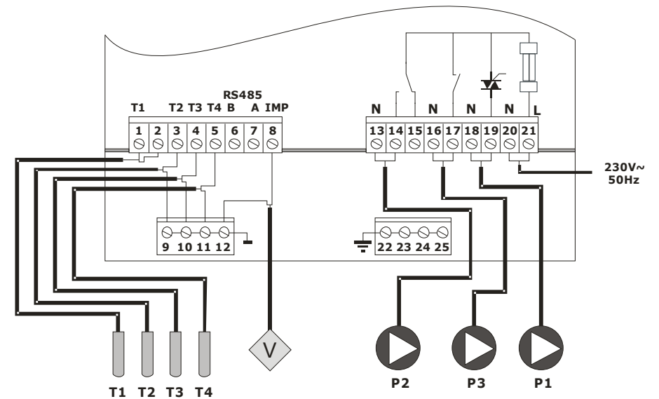
Ilustracja 5: Przykładowy schemat podłączenia
