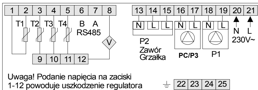
Ilustracja 4: Opis wyprowadzeń
