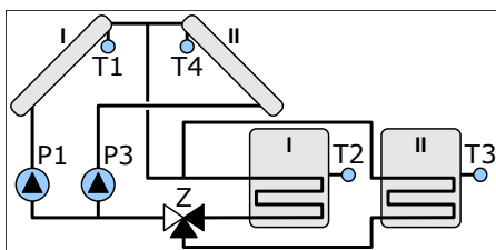
Schemat 11 Ładowanie dwóch zasobników z dwupołociowego układu kolektorów. Sterowanie pracą dwupompowej grupy solarnej. Wybór ładowanego zasobnika za pomocą zaworu rozdzielającego.
