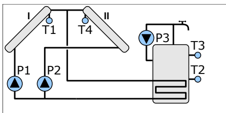
Schemat 12 Ładowanie zasobnika z dwupołociowego układu kolektorów. Sterowanie pracą dwupompowej grupy solarnej. Sterowanie pompą cyrkulacyjną.
