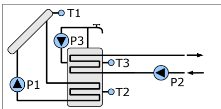
Schemat 4 Ładowanie zasobnika z kolektora słonecznego schemat z trzema czujnikami. Sterowanie pompą cyrkulacyjną. Sterowanie zrzutem nadmiaru ciepła z zasobnika.
