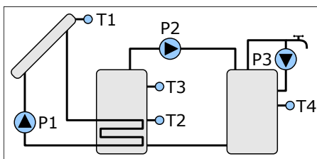
Schemat 5 Ładowanie zasobnika z kolektora słonecznego schemat z trzema czujnikami. Sterowanie pompą cyrkulacyjną. Przepompowywanie ciepła do drugiego zbiornika (na zasadzie różnicy temperatur).
