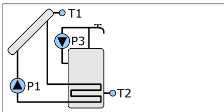
Schemat 1 Ładowanie zasobnika z kolektora słonecznego schemat z dwoma czujnikami. Sterowanie pompą cyrkulacyjną.
