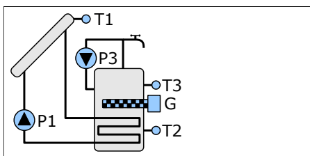
Schemat 3 Ładowanie zasobnika z kolektora słonecznego schemat z trzema czujnikami. Sterowanie pompą cyrkulacyjną. Dogrzewanie zasobnika grzałką.
