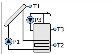
Schemat 2 Ładowanie zasobnika z kolektora słonecznego schemat z trzema czujnikami. Sterowanie pompą cyrkulacyjną.
