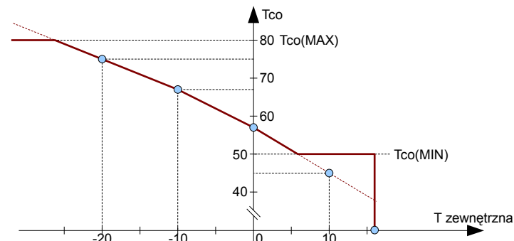
Rysunek 1: Przykładowa charakterystyka grzewcza
