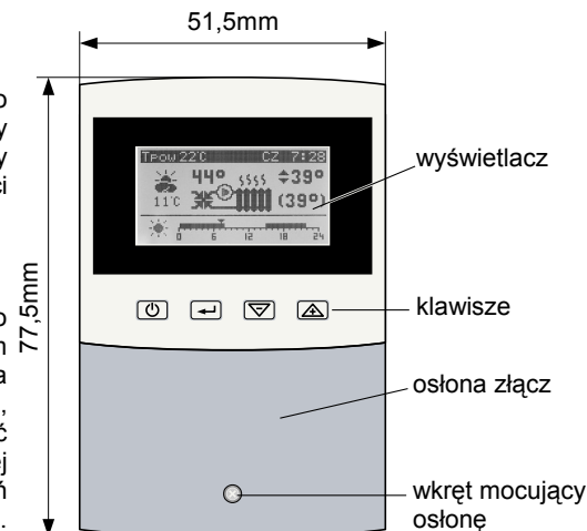
Rysunek 8: Budowa i wymiary termostatu R810.
