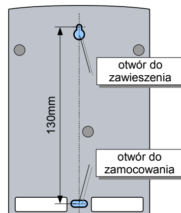
Rysunek 9: Rozmieszczenie otworów montażowych
