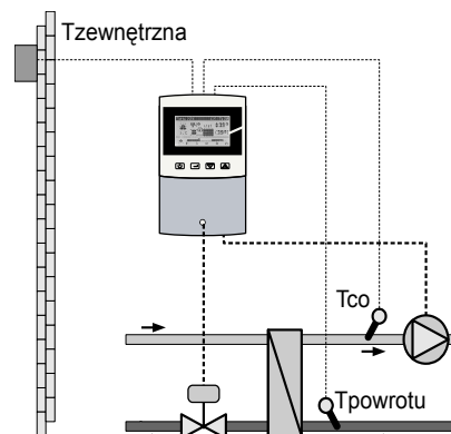
Rysunek 3: Ochrona powrotu z zaworem 2-drogowym.
