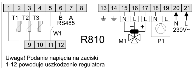
Rysunek 10: Rozmieszczenie wyprowadzeń R810.
