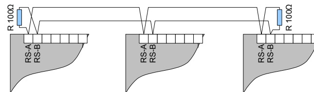
Rysunek 6: Przykładowy schemat prawidłowego połączenia interfejsu RS485
