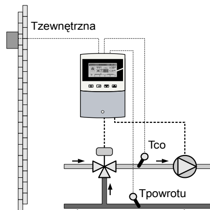
Rysunek 4: Ochrona powrotu zaworem 3-drogowym.
