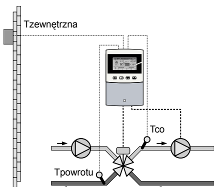
Rysunek 5: Schemat instalacji z zaworem 4-drogowym.
