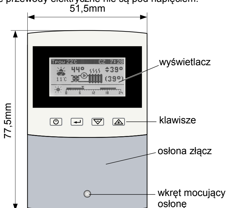
Rysunek 8: Budowa i wymiary termostatu R810.
