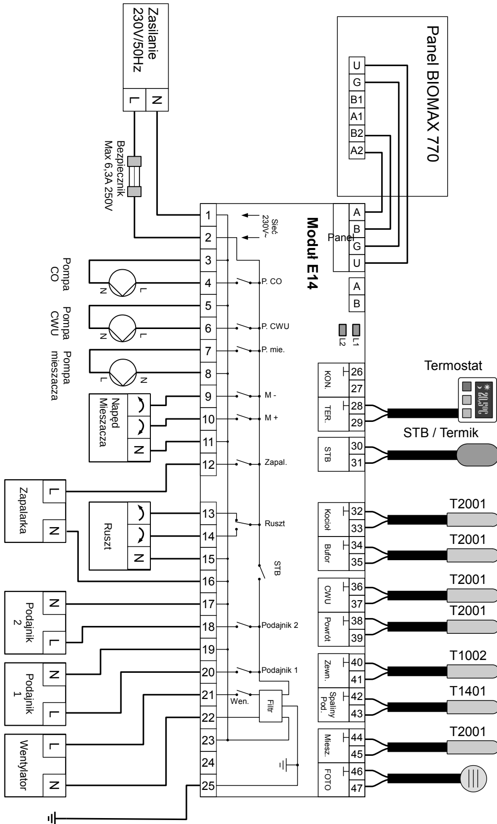
Rysunek 4: Rozmieszczenie wyprowadzeń modułu BIOMAX E14.
