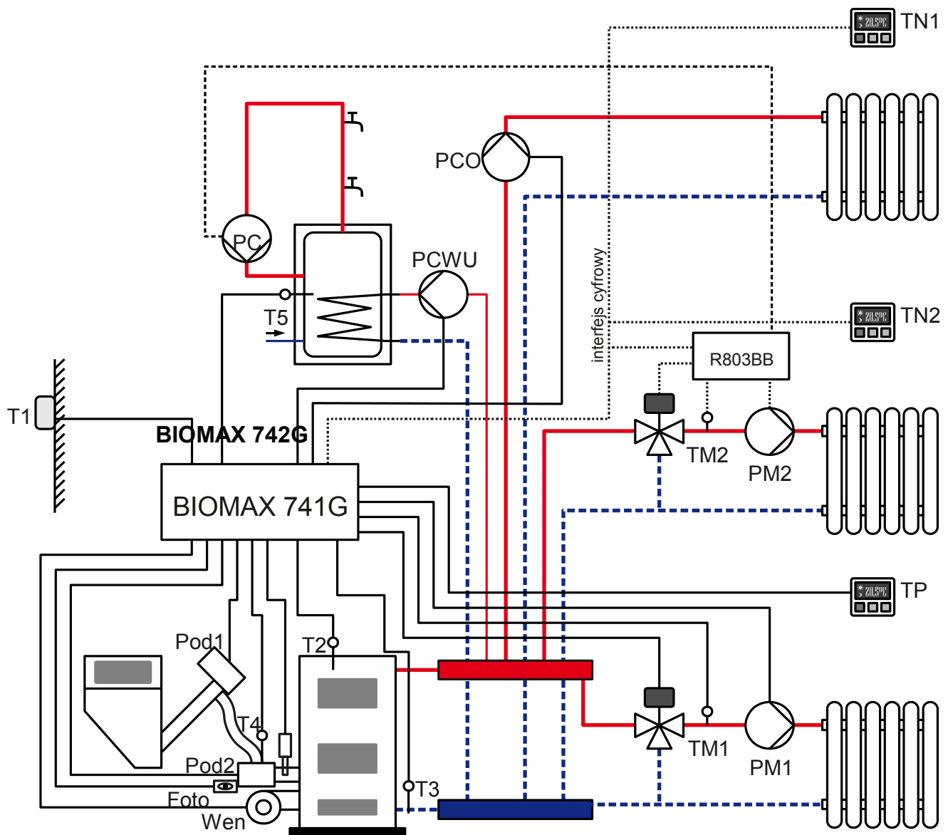
Rysunek 1: Typ instalacji = układ pompowy
