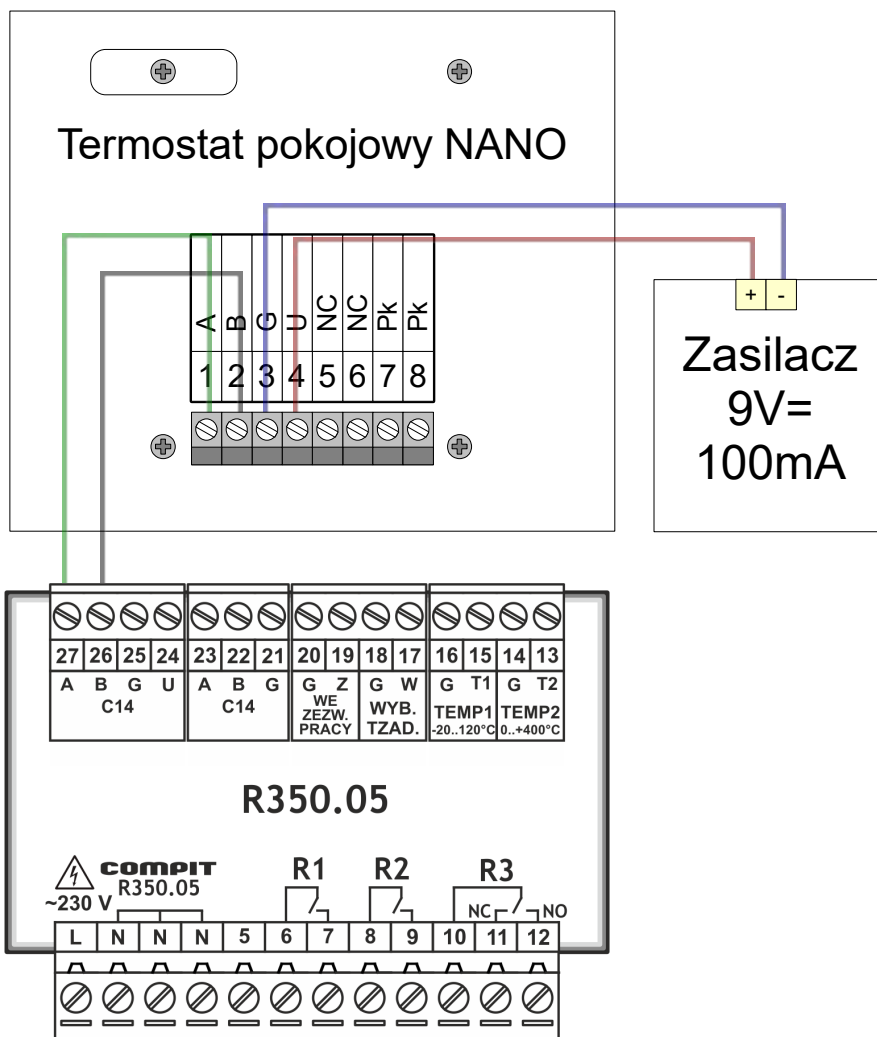
Rysunek 5: Schemat podłączenia R350.05 do regulatora pokojowego NANO.
