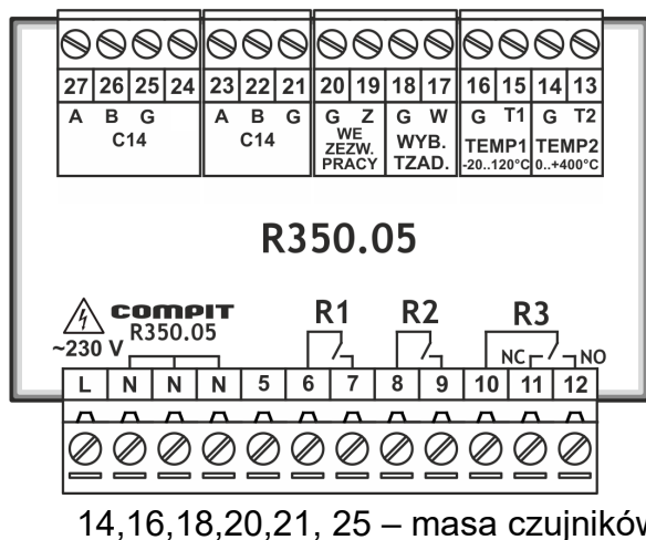
Rysunek 3: Rozmieszczenie wyprowadzeń R350.05.
