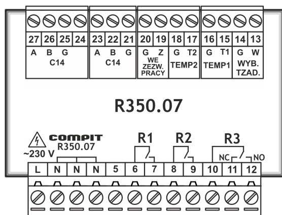
Rysunek 3: Rozmieszczenie wyprowadzeń R350.07.
