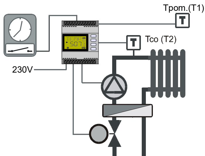
Ilustracja 1: Stabilizacja temperatury pomieszczenia ogrzewanego obiegiem grzewczym o regulowanej temperaturze.
