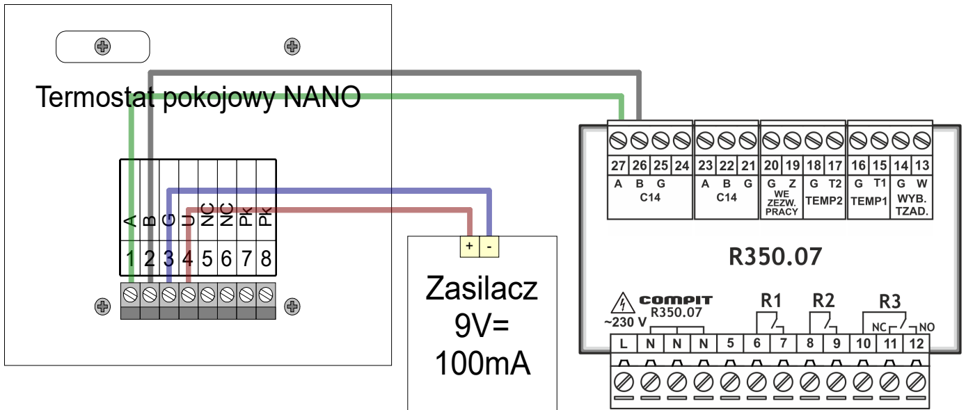
Rysunek 5: Schemat podłączenia R350.07 do regulatora pokojowego NANO.
