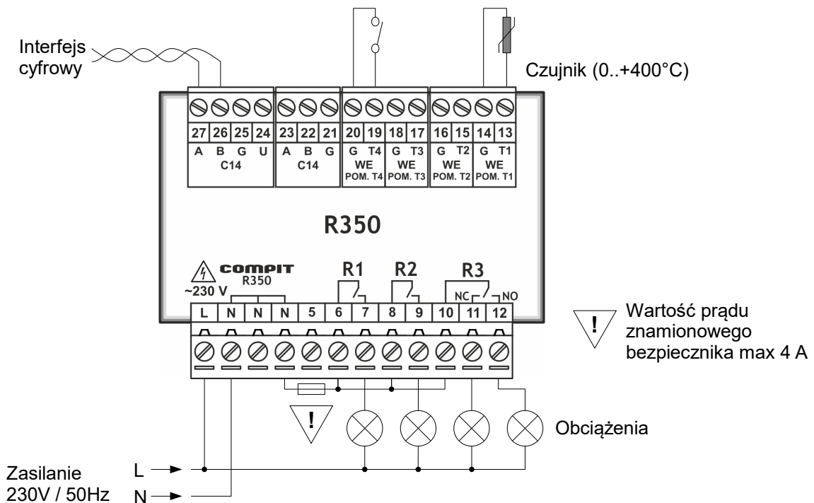
Rysunek 8: Sygnalizacja przekroczenia progów temperatury
