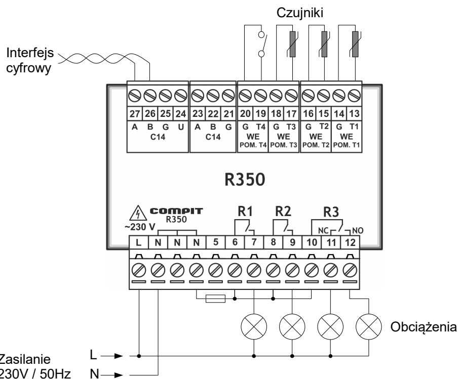
Rysunek 13: Przykładowy schemat sygnalizacji przekroczenia temperatury.
