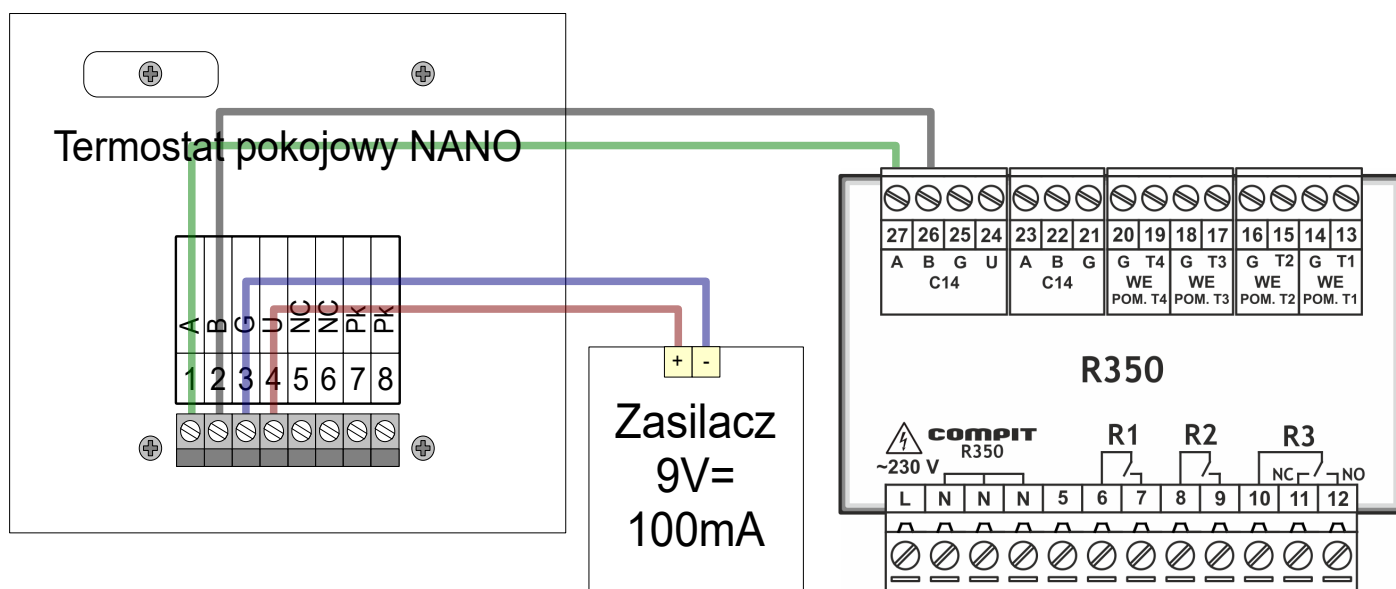
Rysunek 15: Schemat podłączenia R350 do termostatu pokojowego NANO.
