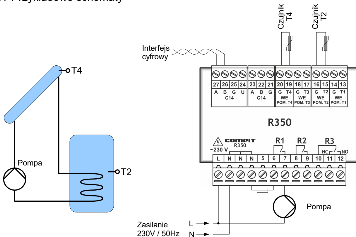
Rysunek 11: Przykładowy sposób zastosowania R350 do sterowania układem solarnym.
