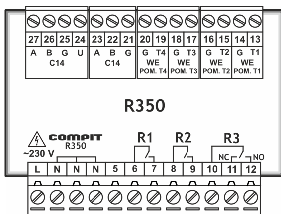
Rysunek 2: Rozmieszczenie wyprowadzeń R350.
