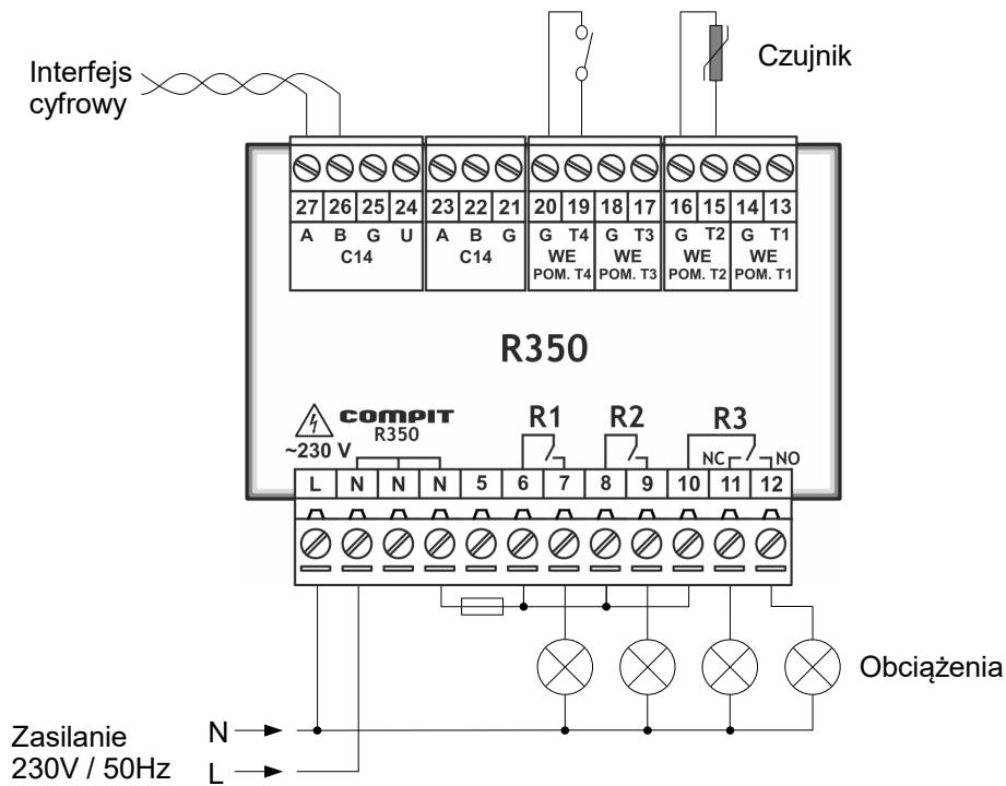
Rysunek 6: Sygnalizacja przekroczenia progów temperatury
